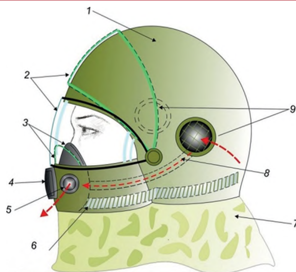
Рисунок 9 – Конструкция универсального «противогаз-бронешлема»: 1 – защитный шлем; 2 – прозрачное забрало; 3 – носогубный эластичный экран; 4 – переговорное устройство; 5 – выдыхательный клапан; 6 – линия обтюрации; 7 – защитная пелерина шеи; 8 – внутренние воздуховоды для подачи выдыхаемого воздуха от фильтрующе-сорбирующих элементов внутрь экрана; 9 – фильтрующие (сорбирующие) сменные фильтры суточного действия (рисунок подготовлен авторами по [15])
