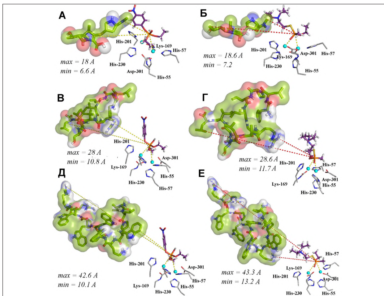
Рисунок 6 – Модели молекулярного взаимодействия параоксона (А, В, Д) и вещества ви-икс (Б, Г, Е) с активным центром фермента His 6 -ОРН при pH 7,5 в присутствии меропенема (А, Б), темпорина А (В, Г), и индолицидина (Д, Е). Молекулы ФОС представлены фиолетовым цветом, антибиотики – зеленым. Ключевые аминокислотные остатки активного центра и ионы Co 2+ окрашены в серый и голубой цвет соответственно.
