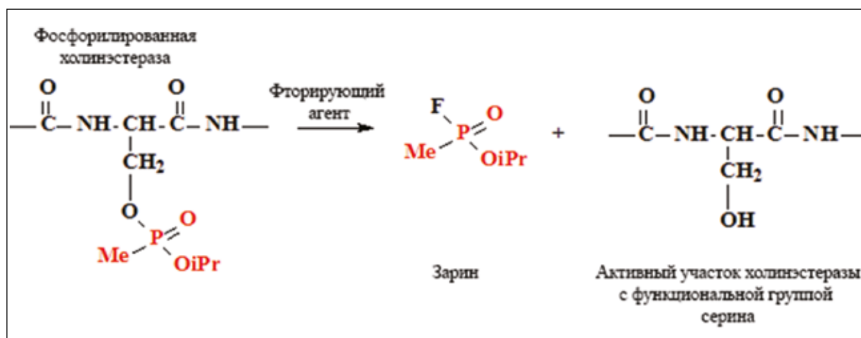
Рисунок 4 — Схема реакции обработка фосфорилированной холинэстеразы фторирующим агентом
