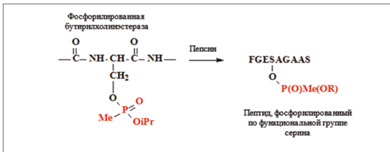
Рисунок 5 — Схема реакции обработки фосфорилированной бутирилхолинэстеразы пепсином
