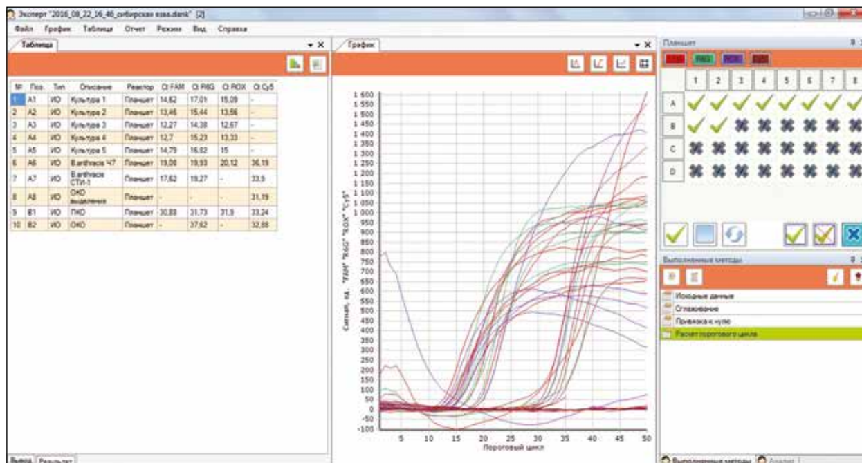
Рисунок 4 — Результаты исследования выделенных микробных культур методом ПЦР-РВ
