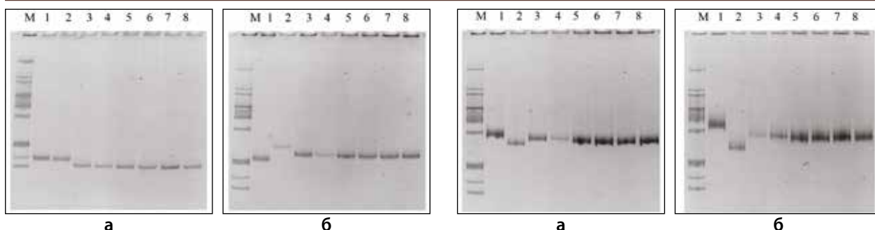
Рисунок 11 — Электрофореграмма фракционирования в 8 % ПААГ продуктов амплификации VNTR-локусов сибирезвенного микроба Ceb-Bams-3 (а) и Ceb-Bams-13 (б) (М – молекулярный маркер ДНК GeneRuler™ 100 br DNA LadderPlus; 1–8 – продукты амплификации локусов Ceb-Bams-3 (а) и Ceb-Bams-13 (б): 1 – СТИ-1, 2 – Ч-7; 3 – 1051; 4–8 – выделенные из проб микробные культуры B. anthracis )
